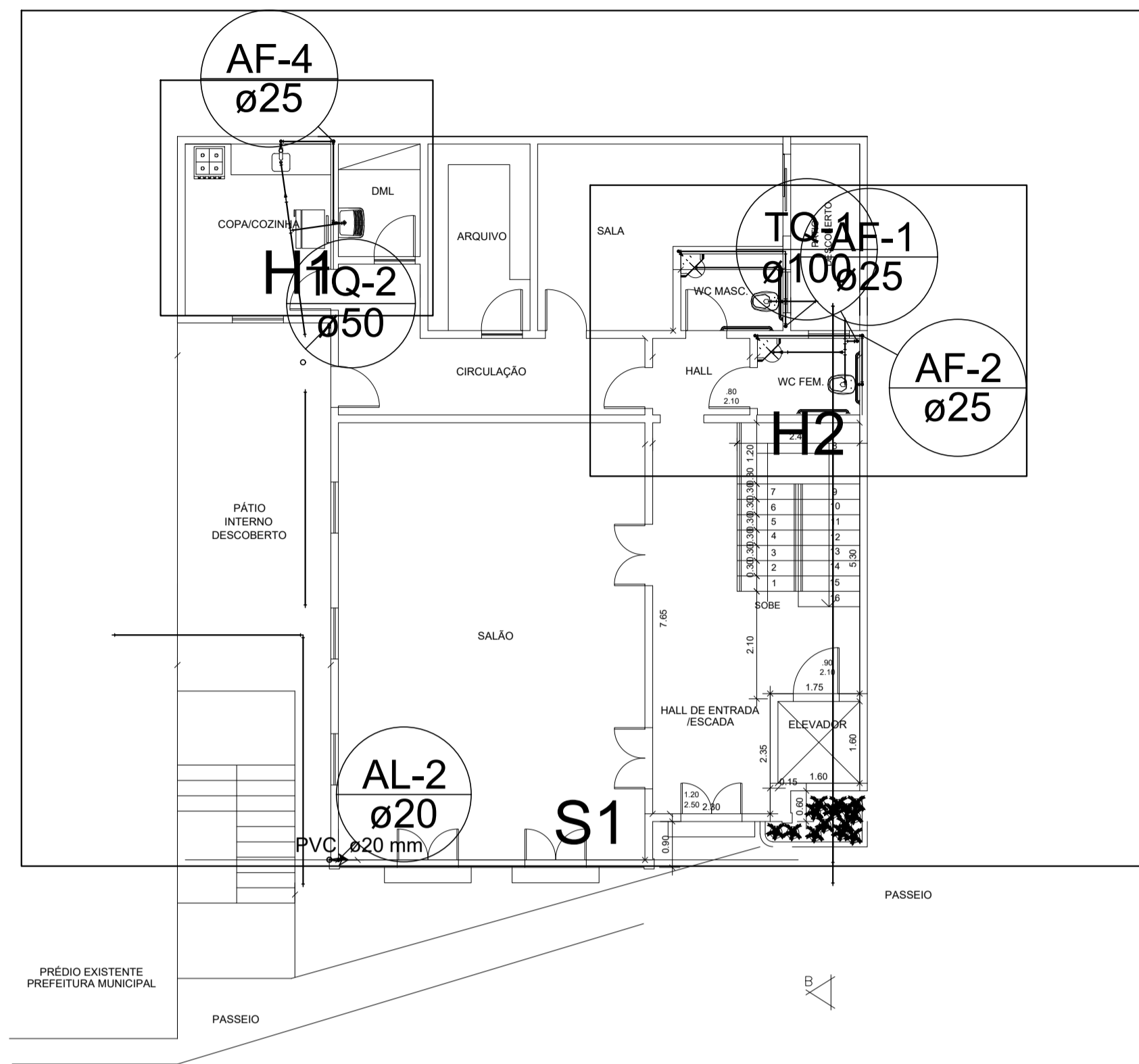
1 PLANTA BAIXA / TÉRREO ESCALA: 1/75
