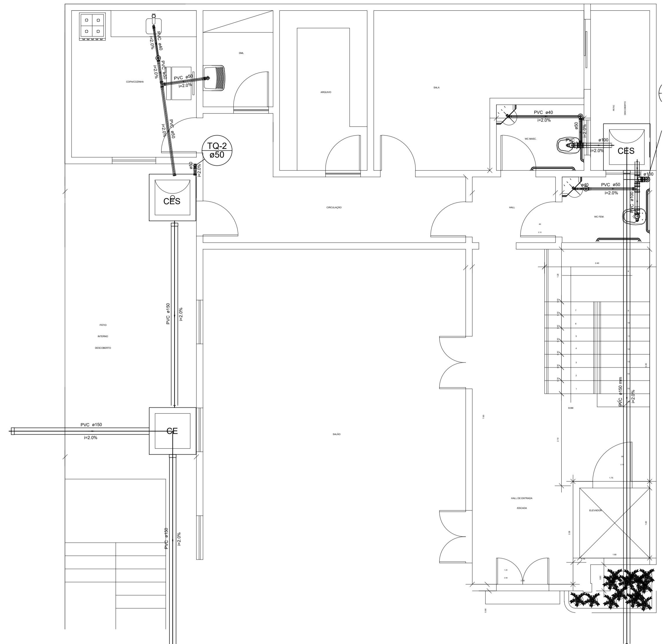
Detalhe S3 escala 1:50
